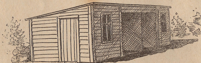
Podoba šte. 5. Perotninski hlev za dva plemena.
